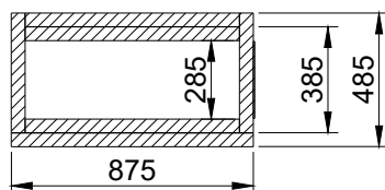
B-B (1:30)
