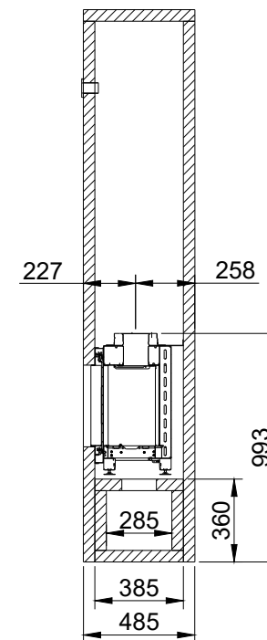
D-D (1:30)
